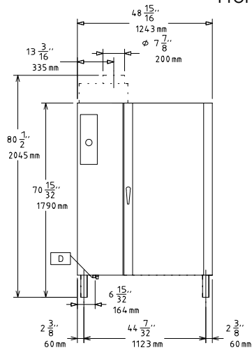
Front aanzicht
